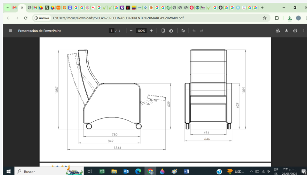
Planos dimensionales — posición normal y reclinada
